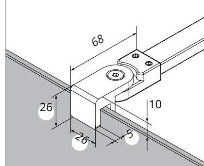
c VINKELRETT BESLAG
