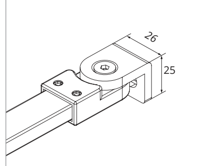
b VINKELRETT BESLAG
